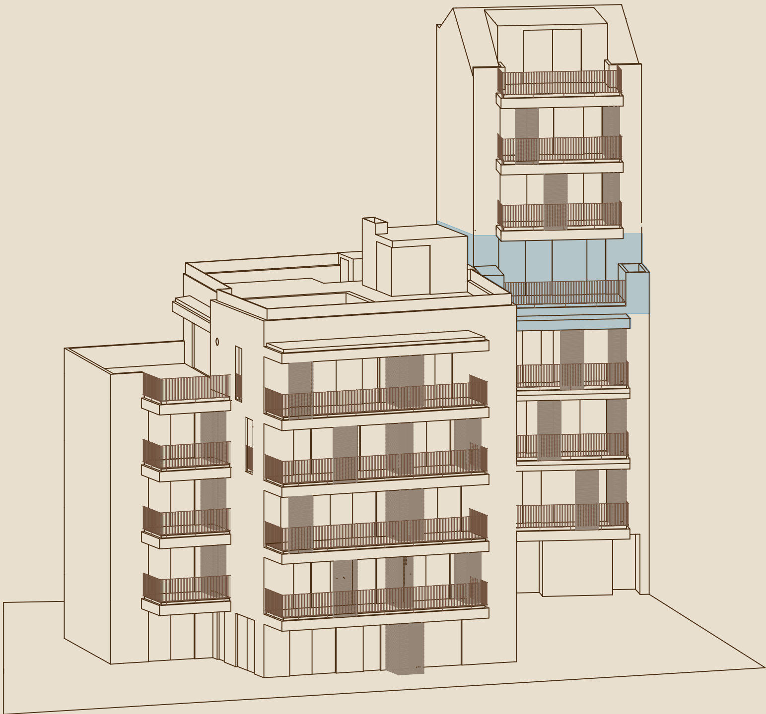
AXONOMETRIA
